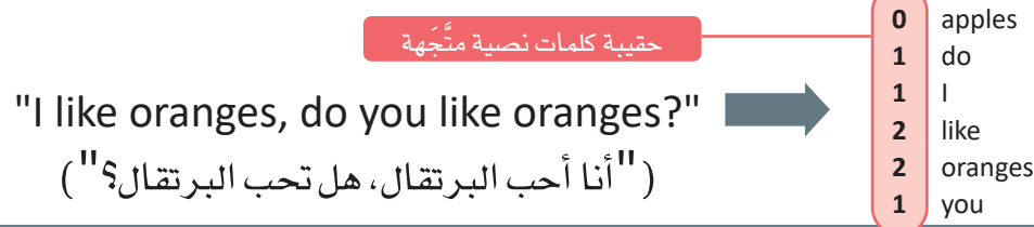
شكل 3.5: تمثيل حقيبة الكلمات (bag-of-words)
