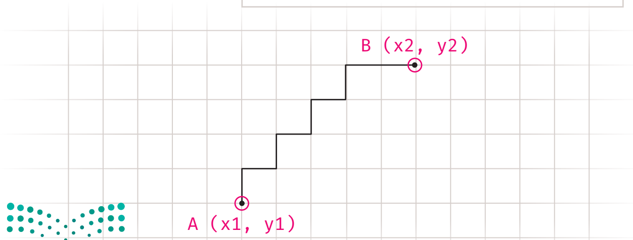
شكل 2.25: مسافة مانهاتن
